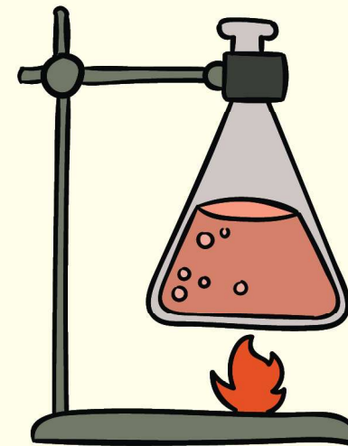
Zat Kimia
